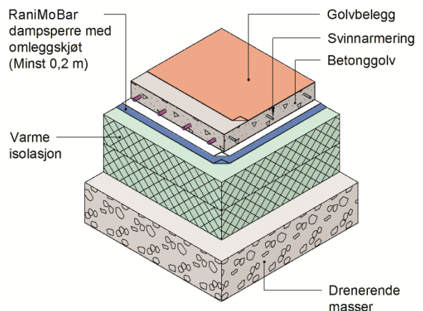
Fig 3 RaniMoBar Dampspærre montert i betonggolv på grunnen
