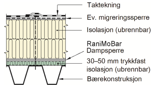
Fig. 1 RaniMoBar Dampspærre montert i kompakt takkonstruksjon
