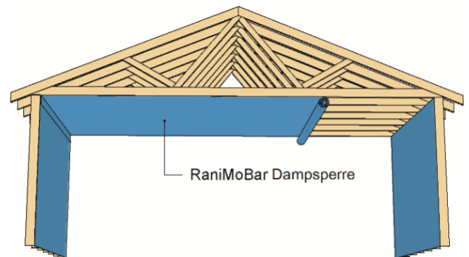
Fig. 2 RaniMoBar Dampspærre montert i yttervegger og mot kaldt loftsrom
